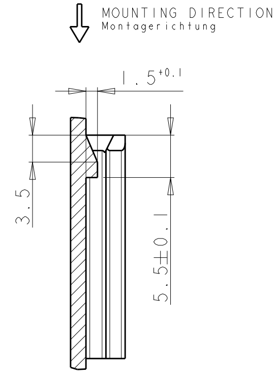
SECTION A-A Schnitt
