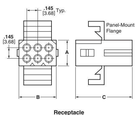
Receptacle
