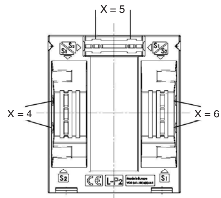
Anschlussbelegung
