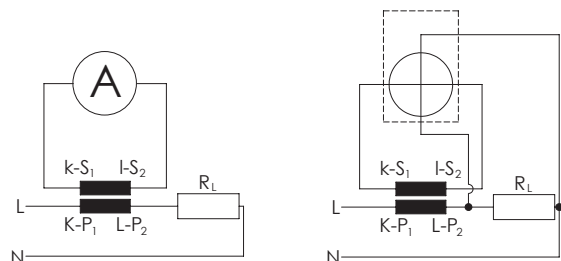
Meßschaltung
