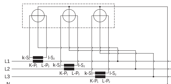
Zählerschaltung mehrphasig
