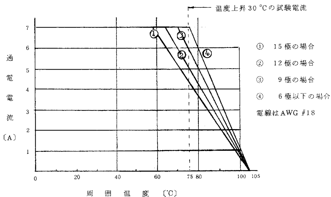
図 1 周囲温度—通電電流特性
