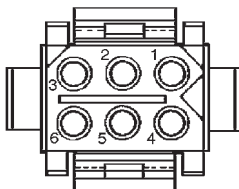
Receptacle
