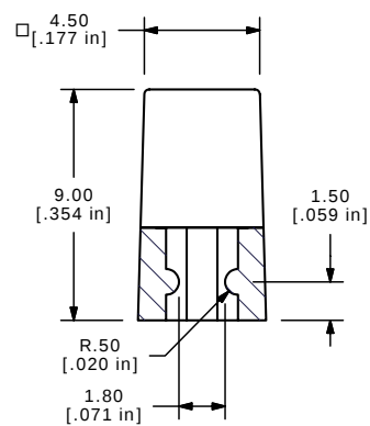
SECTION A-A SCALE 4 : 1
