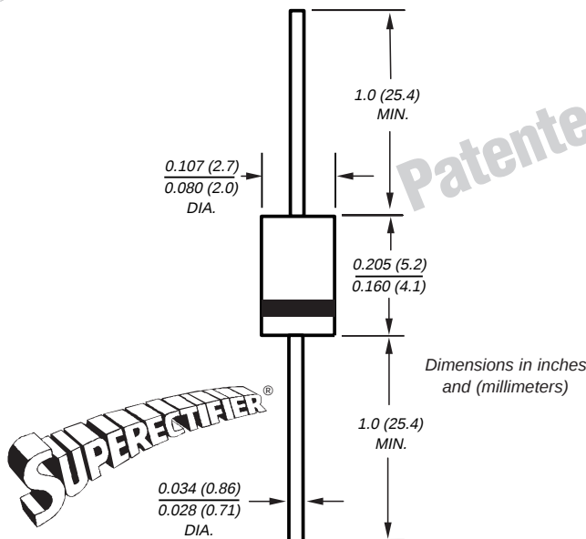
DO-204AL (DO-41)
