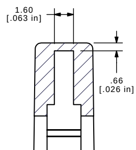
SECTION B-B SCALE 4 : 1
