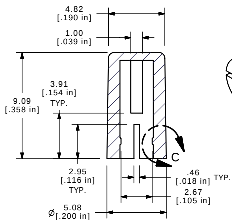
SECTION A-A SCALE 4 : 1
