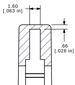
SECTION B-B SCALE 4 : 1
