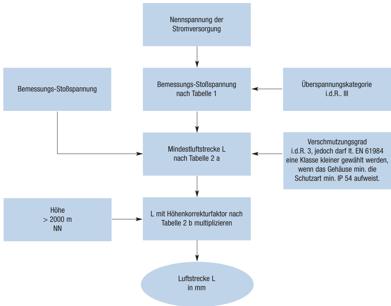
Schema zur Ermittlung der Luftstrecken
