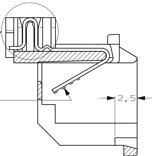
SEC. A-A
