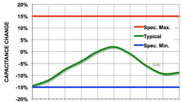
BME MINI SWITCHMODE TEMPERATURE COEFFICIENT
