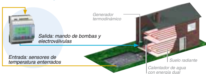
Control de calefacción y gestión de agua caliente sanitaria: bomba de calor
