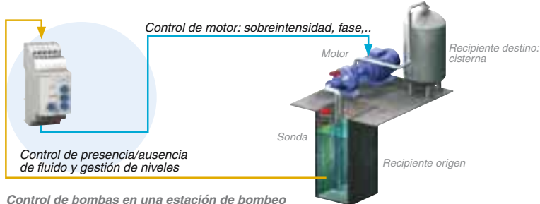
Control de bombas en una estación de bombeo
