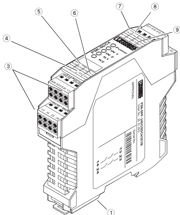
PSR-SPP- 24DC/SDC4/2X1/B
