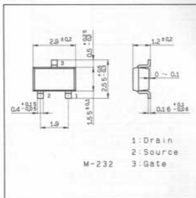
外形寸法図
