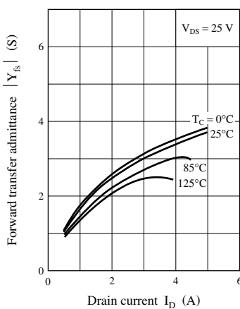
|Y_{fs}| - I_D
