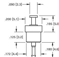
Feed-Thru
