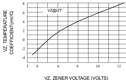
Fig. 2-ZENER VOLTAGE-TO 12 VOLTS
