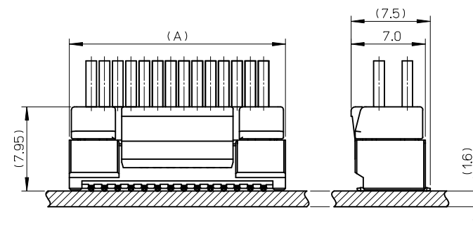
嵌合状態図 MATED CONNECTORS
