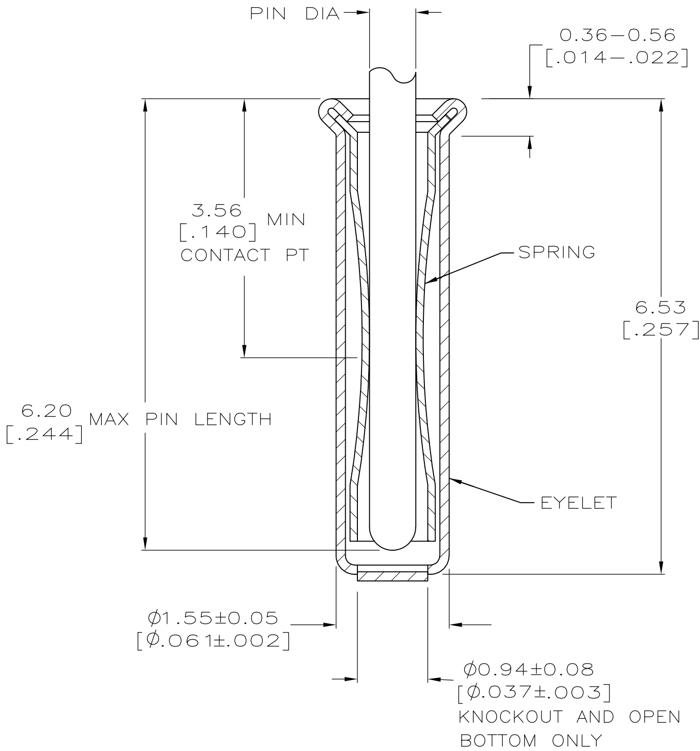
SECTION A-A
