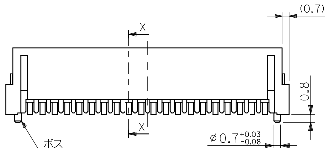
嵌合図 MATING REC.
