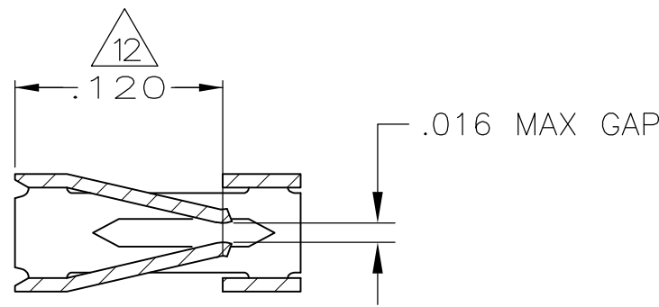
SECTION D-D
