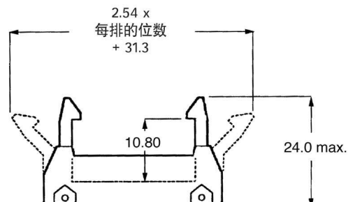
低型面闭锁 (型号 2)
