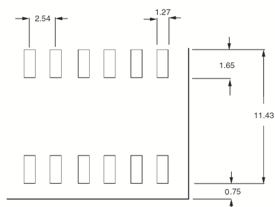
推荐的 PCB 布局
