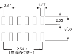
推荐的 PCB 布局
