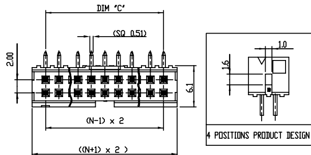
10072354 Right angle
