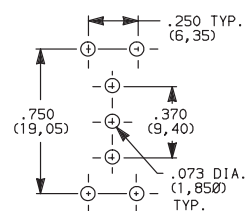
7101J1_BE2 SPDT
