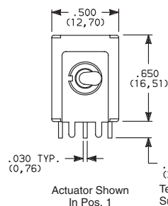
7301MD9ABE Horizontal Actuation 3PDT
