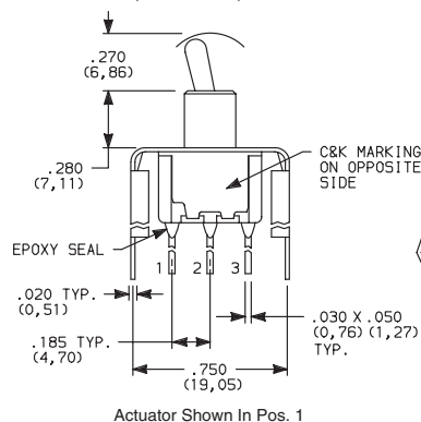
7101MD9_BE SPDT
