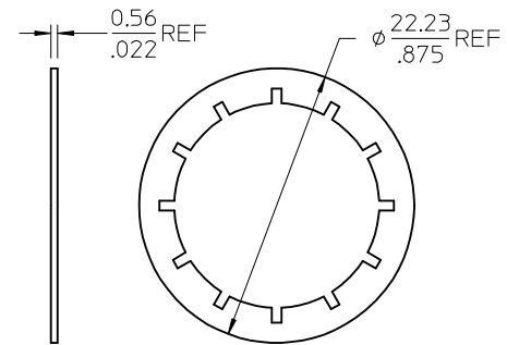
LOCKWASHER
