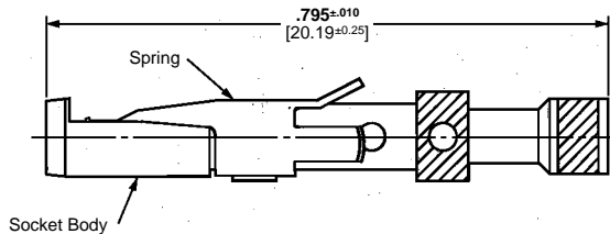
Socket
