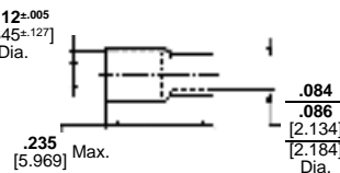
Ferrule
