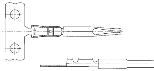
Socket
