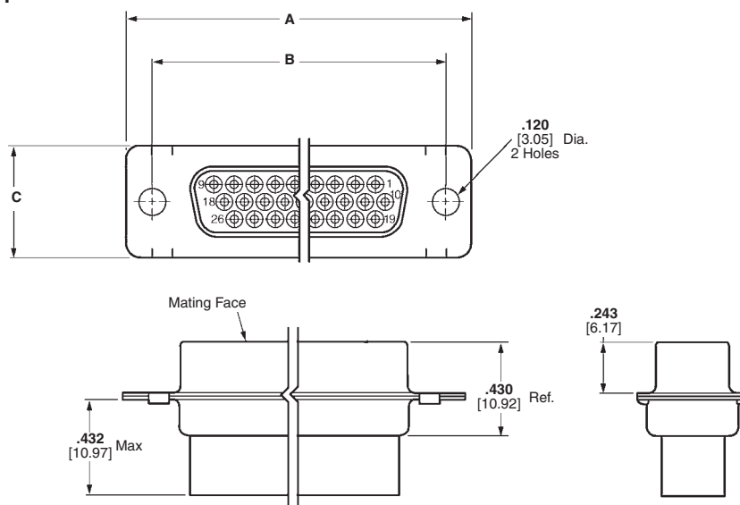
Receptacle
