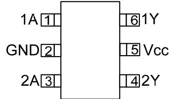
SOT363
