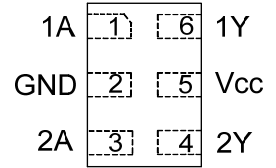
X2-DFN1410-6
