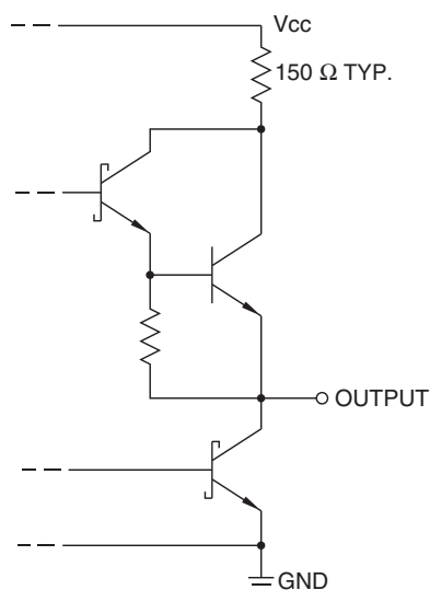
74OL6000/01 Output
