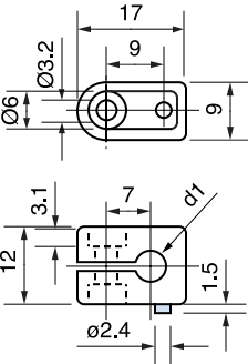
Flange for Ø4 - M5 - Ø6.5
