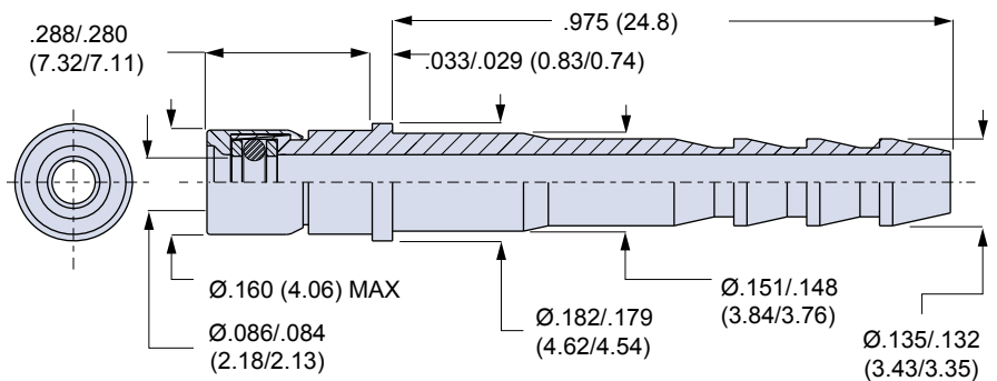
830-004 Socket Contact
