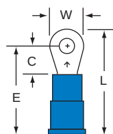
12-4S-P Stud Size 4 Wire Range 16-14
