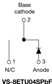
VS-8ETU04SPbF
