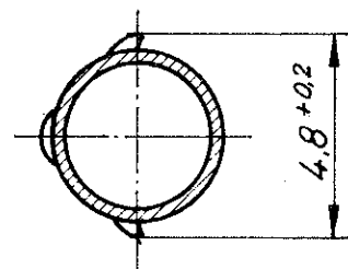
Schnitt: D - D
