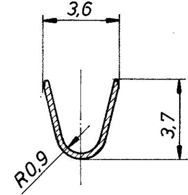
Schnitt: C - C
