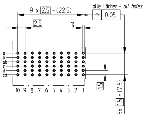
Lochbild für Leiterplatte (Bestückungsseite)
