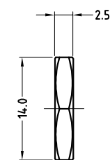
METAL NUT
