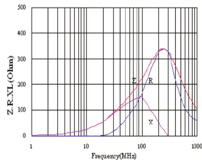
ACML-0805-221
