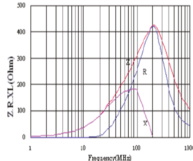
ACML-0805-152
