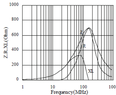
ACML-0805-601
