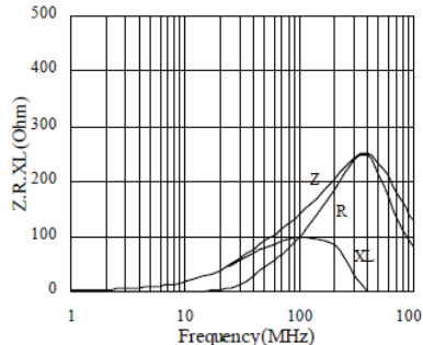
ACML-0805-151
