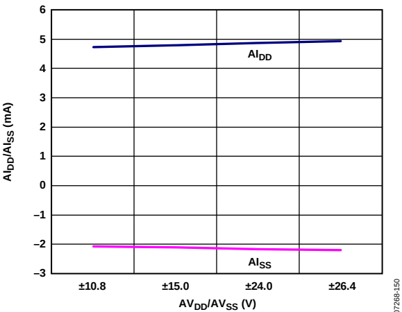
Figure 50. A IDD /A ISS vs. AV DD /AV SS , I OUT = 0 mA
