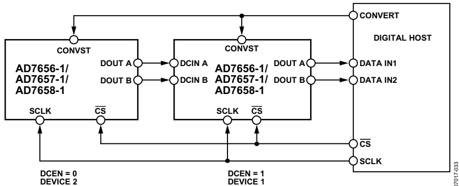
图36. 菊花链配置
