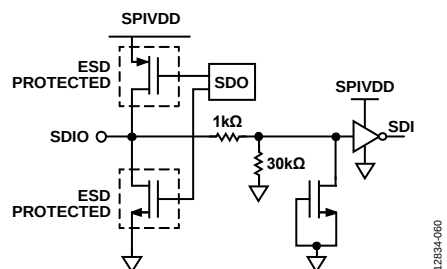
Figure 60. SDIO Input
