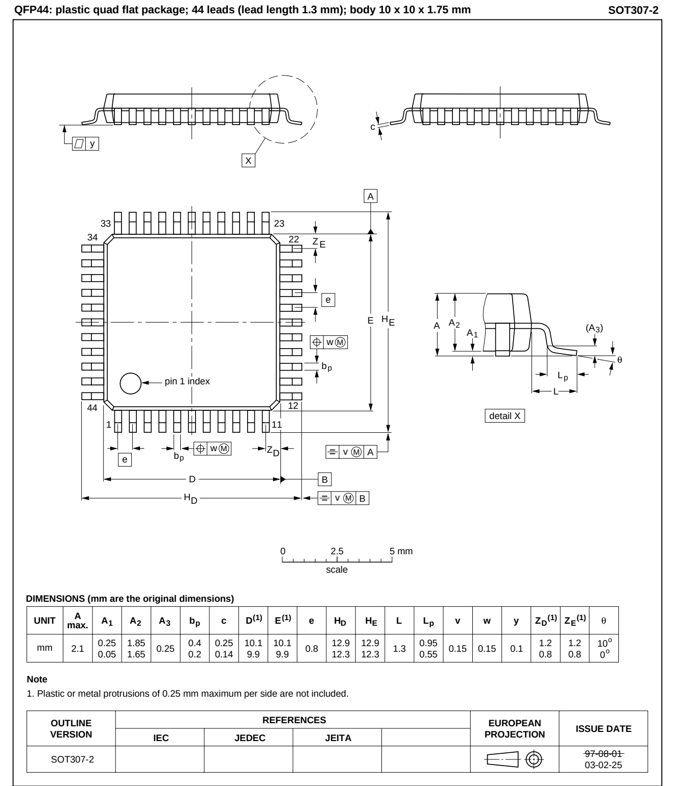
Fig 28. SOT307-2 (QFP44)
