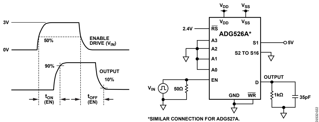
Figure 22. Enable Delay, t_{ON}(EN) t_{OFF}(EN)
