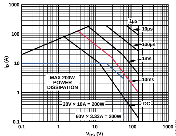
Figure 49. FET SOA
