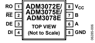
Figure 6. ADM3072E/ADM3075E/ADM3078E Pin Configuration
