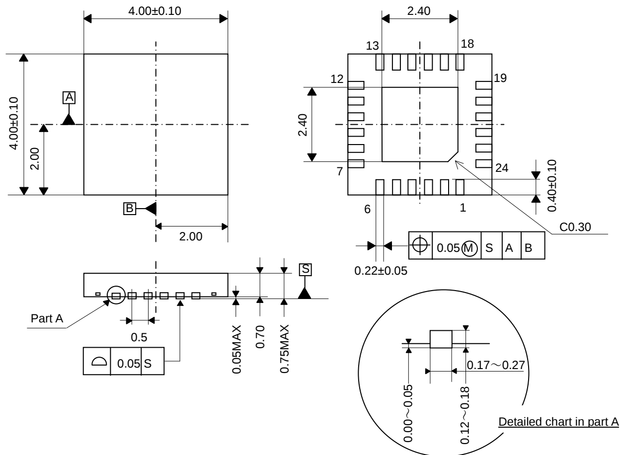
Fig. 16 Outer Dimensions
