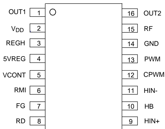
TSSOP-16
