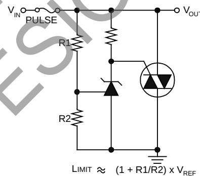
Fig. 9 Crow Bar
