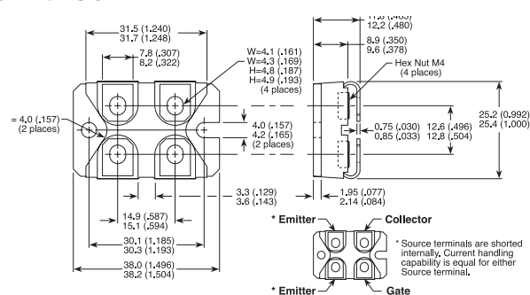
ISOTOP ® or SOT-227
